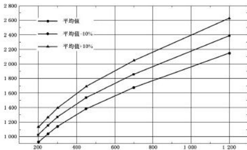
b) 簾布袋冲击试验垂直微应变参考平均峰值
